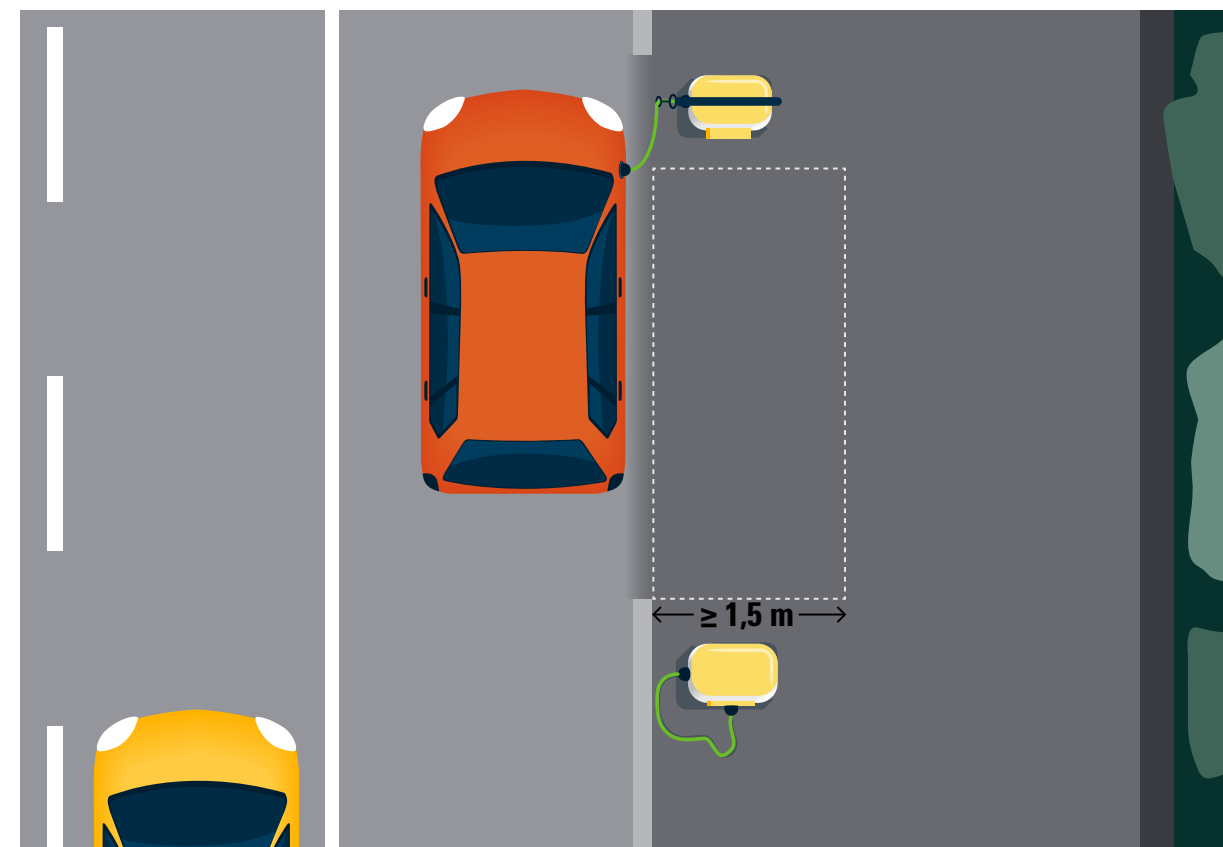
Abbildung 5.4: Ladeplatz in Längsaufstellung mit unverbaute angrenzender Fläche von 1,50 m Breite (rechts)
