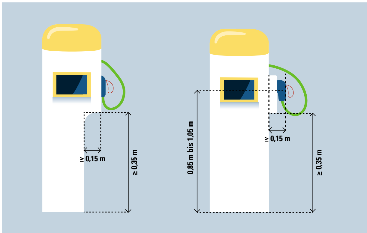
Abbildung 5.1: Unterfahrbarkeit
