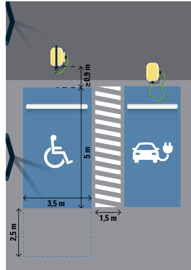
Abbildung 5.5: Ladeplatz Anfahrbarkeit
